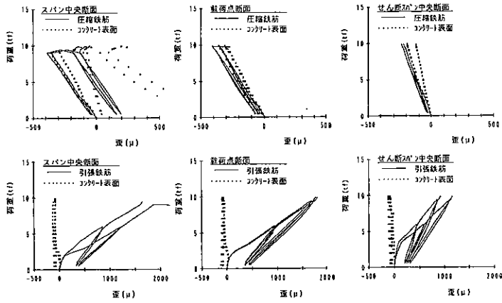
図-16 (a) 鉄筋及びコンクリート表面ひずみの関係 (在来合板型枠によるRCはり)
