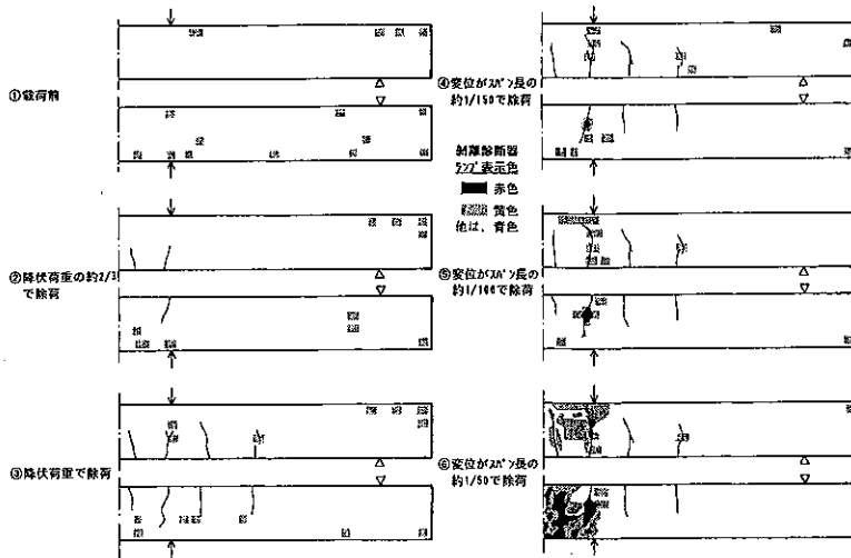
図-17 (a) 剝離診断器による GRC 型枠の剝離状況 (凸凹内面 GRC 型枠による RC はり)
