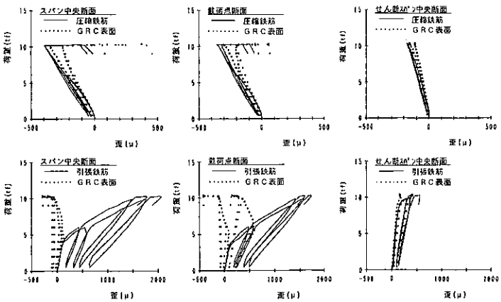
図-16 (c) 鉄筋及びコンクリート表面ひずみの関係 (金網埋込内面 GRC 型枠による RC はり)
