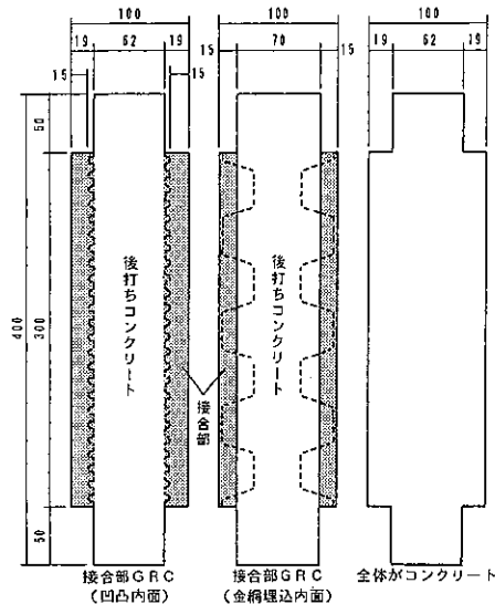
図-4 部分圧縮試験体の形状寸法
