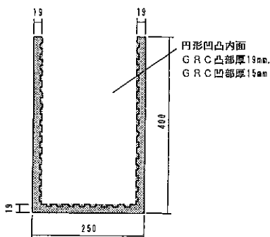
図-2 円形凸凹内面 U 字型一体成型型枠
