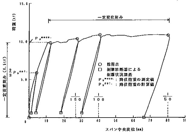
図-8 GRC 打込み型枠を用いた RC はりの X-Y レコーダによる荷重—変位曲線
