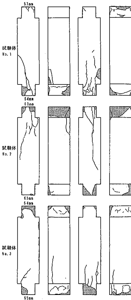
図-11 (a) 部分圧縮試験体の最終ひび割れ破壊状況 (全体がコンクリート, 現場封緘養生)
