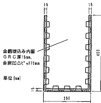
図-3 金網埋込み内面 U 字型組立成型型枠
