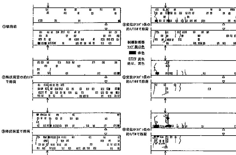
図-17 (b) 剝離診断器による GRC 型枠の剝離状況 (金網埋込内面 GRC 型枠による RC はり)
