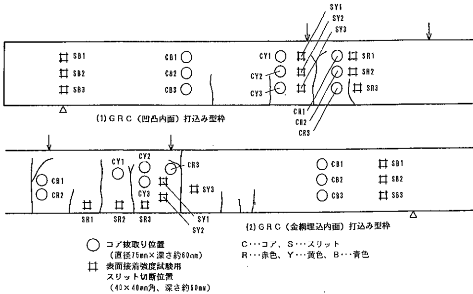
図-18 コア抜き取り及び表面接着強度試験用スリット加工位置
