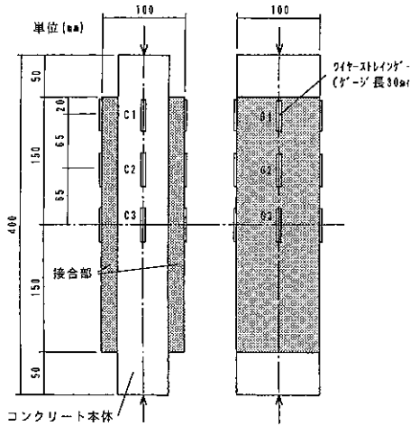
図-5 表面ひずみの測定位置
