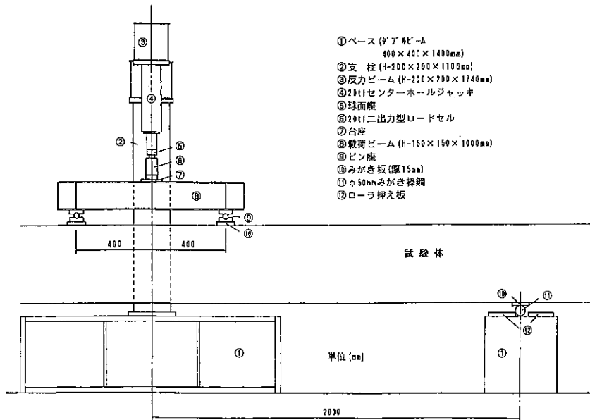
図-7 RC はりの曲げ荷試験
