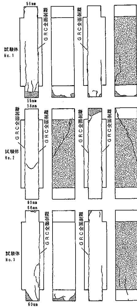
図-11 (b) 部分圧縮試験体の最終ひび割れ破壊状況 (接合部が凸凹内面 GRC 型枠, 現場封緘養生)
