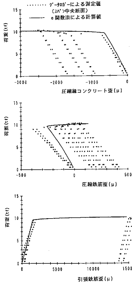
図-15 (a) 荷重—ひずみ関係の測定値と計算値 (在来合板型枠によるRC はり)
