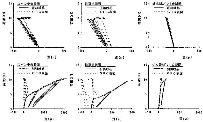
図-16 (b) 鉄筋及びコンクリート表面ひずみの関係 (凸凹内面 GRC 型枠による RC はり)
