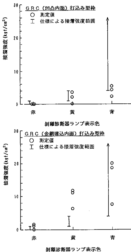
図-19 剝離診断器のランプ表示色と表面接着強度の測定値の対応
