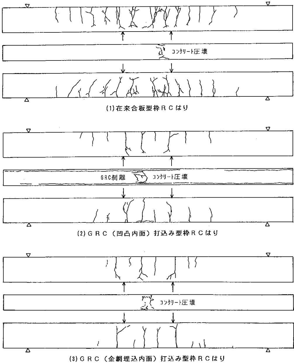
図-13 RC はりの最終的ひび割れ及び破壊状況
