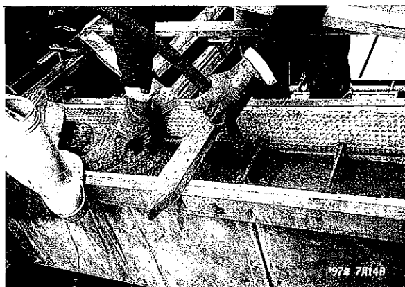
GRC 打込み型枠施工試験
